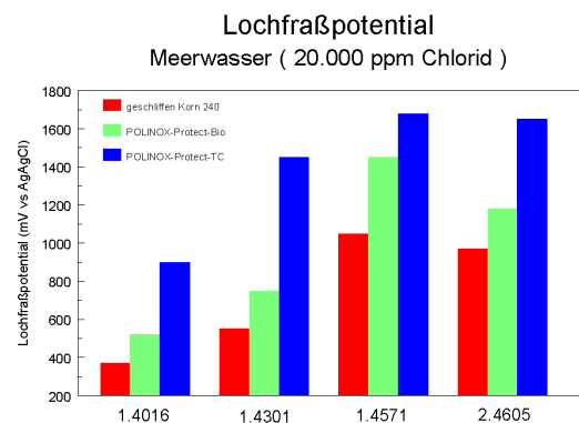
Abb. 3: Lochfraßpotentiale (mV) auf verschiedenen Edelstahl-Qualitäten, Oberfläche geschliffen mit K 240, unbehandelt, POLINOX Protect und POLINOX Protect TC
