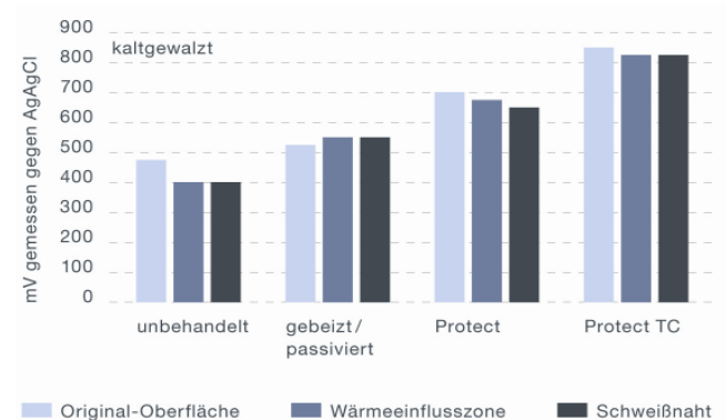
Abb. 5: Korrosionsbeständigkeit im Schweißnahtbereich
