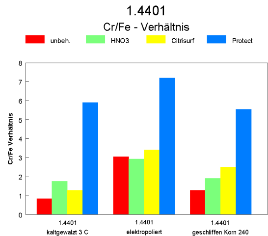
Abb. 1: Chrom-Eisen-Verhältnis auf Edelstahl nach Passivierung mit POLINOX Protect; Quelle: Universität der Bundeswehr, Neubiberg, Institut für Elektrotechnik
